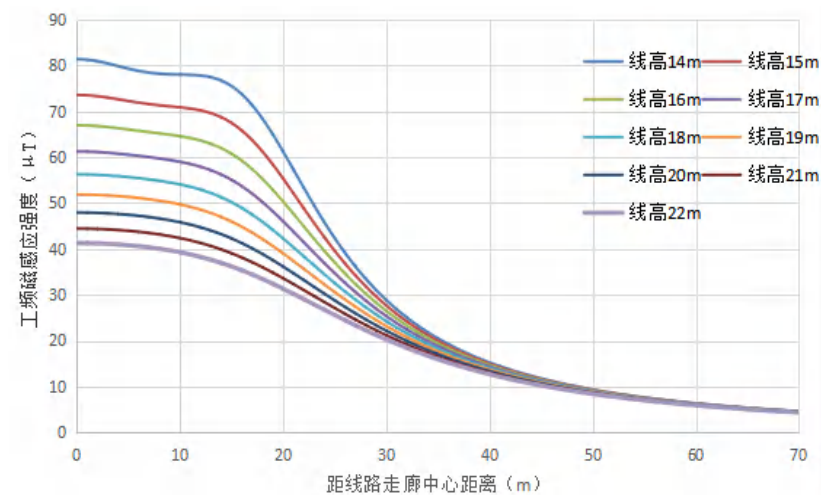
图 6.1-32 单回（水平排列）线路距地面 1.5m 高处工频磁场预测图
