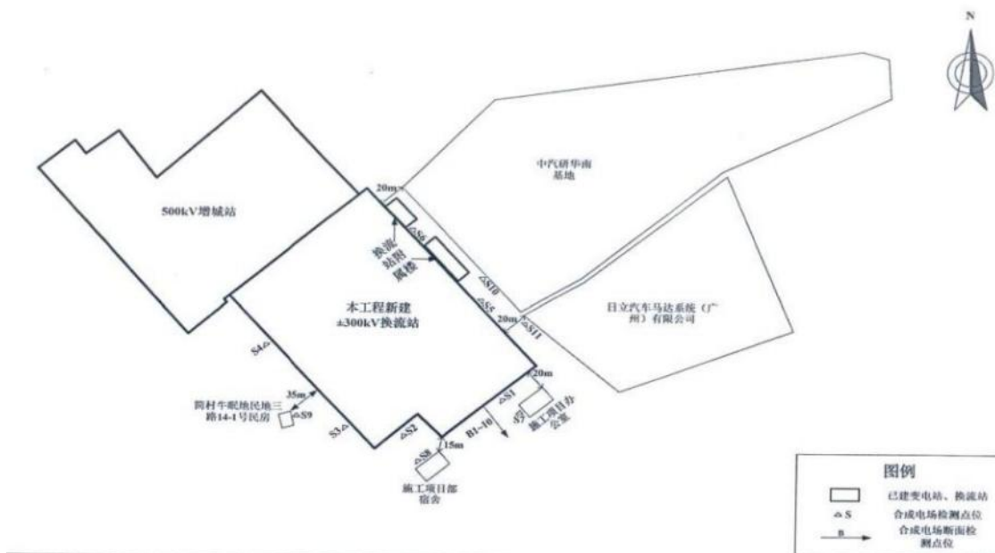
图 6.1-3 类比换流站（中通道换流站）合成电场监测布点示意图
