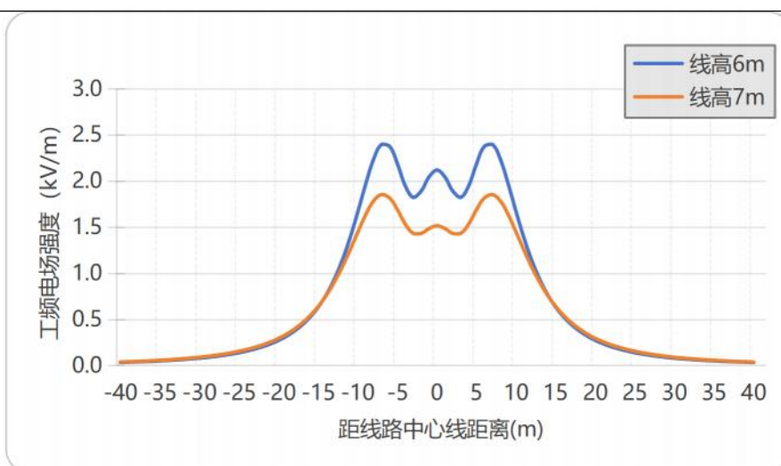
图 6.1-66 水平排列段线路距地面 1.5m 高处工频电场预测图
