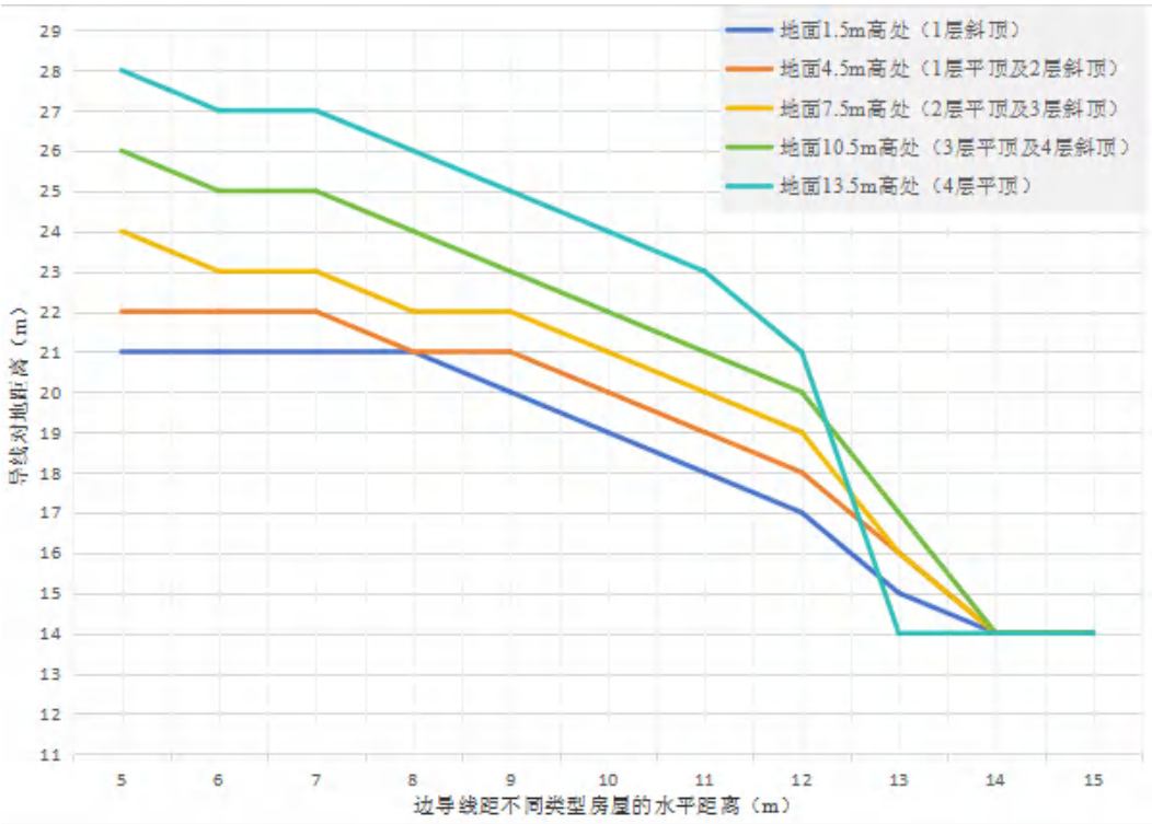
图 6.1-41 单回线路（水平排列）路线不同高度处工频电场强度 4kV/m 等值线图
