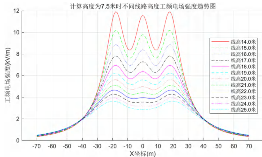
图 6.1-57 20mm 冰区单回水平线路距地面 7.5m 高处工频电场预测图
