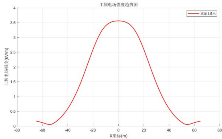
图 6.1-60 15mm 冰区双回共塔线路距地面 1.5m 高处工频电场预测图（线高 27m）
