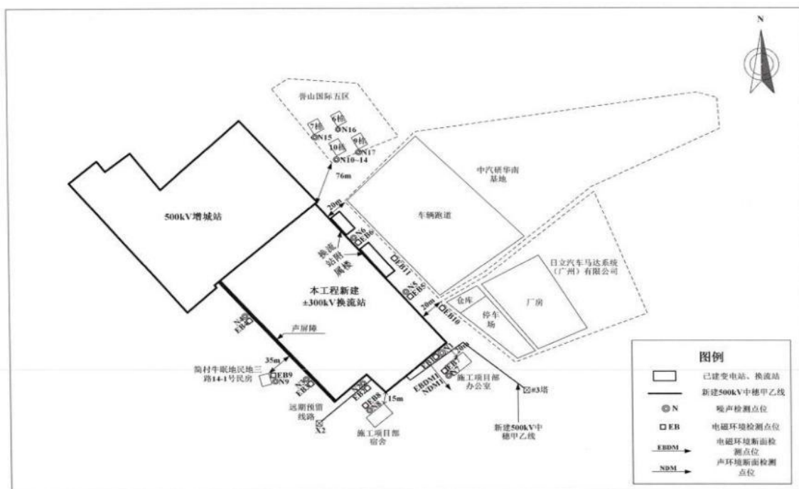
图 6.1-2 类比换流站（中通道换流站）工频电场、工频磁场监测布点示意图
