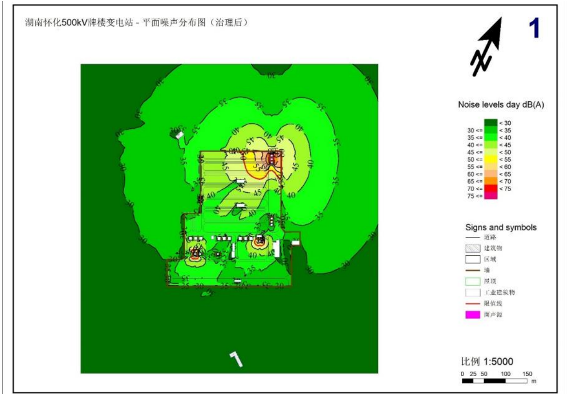
图 6.2-4 牌楼 500kV 变电站本期采取措施后噪声贡献值等值线分布图
