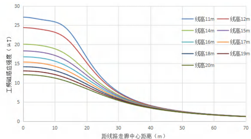
图 6.1-19 单回（水平排列）线路距地面 1.5m 高处工频磁场预测图
