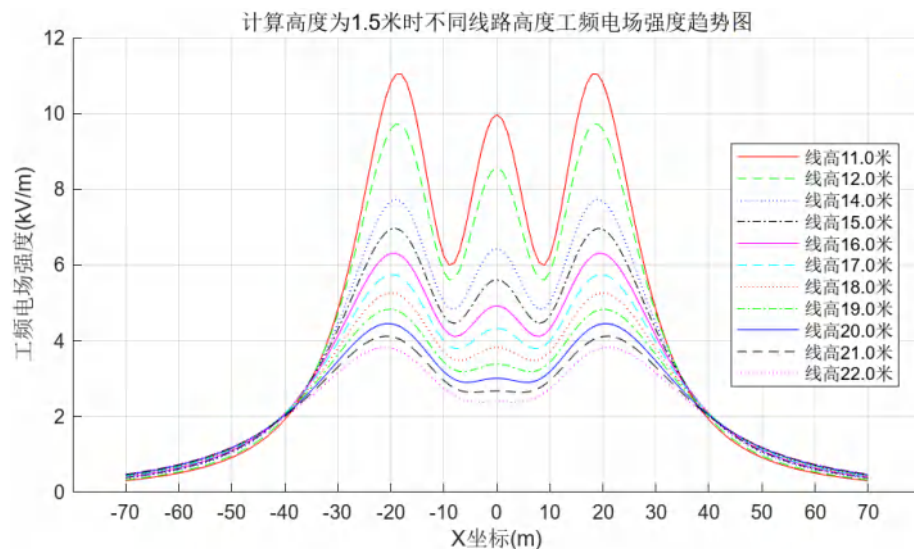
图 6.1-53 20mm 冰区单回水平线路距地面 1.5m 高处工频电场预测图
