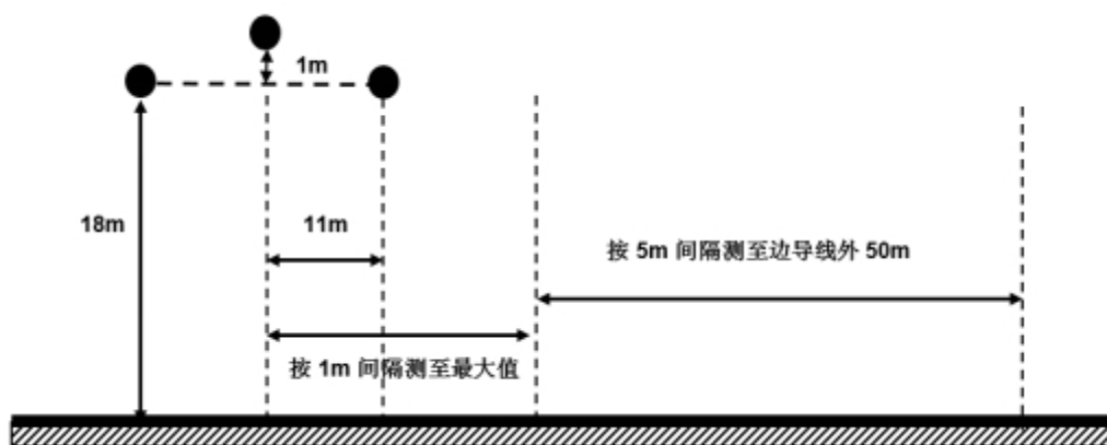
图 6.1-7 500kV 雁船 II 线电磁环境监测断面示意图
