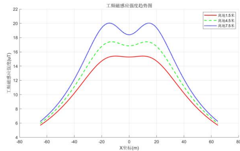
图 6.1-63 15mm 冰区双回共塔线路距地面 1.5m、4.5m、7.5m 高处工频电场预测图（线高 29m）
