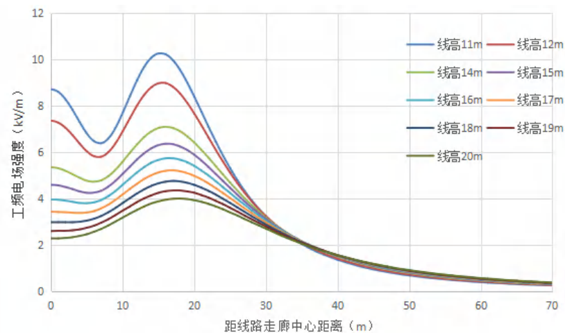
图 6.1-18 单回（水平排列）线路距地面 1.5m 高处工频电场预测图
