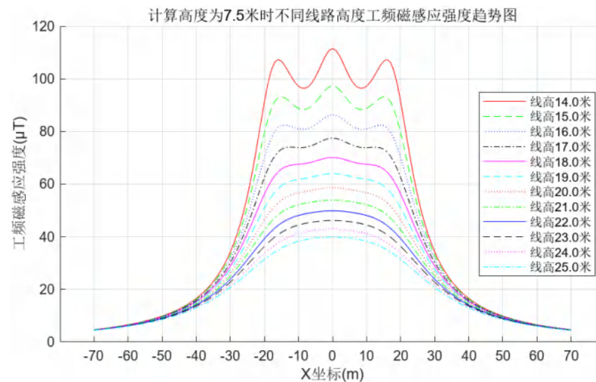
图 6.1-58 20mm 冰区单回水平线路距地面 7.5m 高处工频磁场预测图
