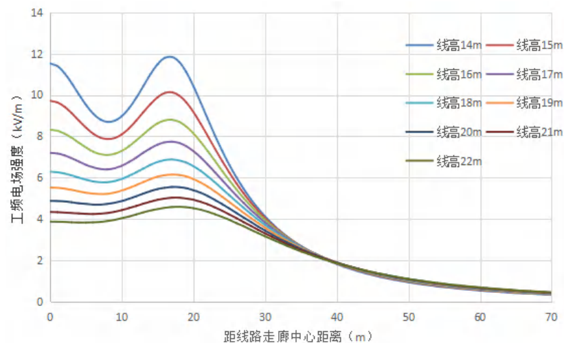
图 6.1-35 单回（水平排列）线路距地面 7.5m 高处工频电场预测图
