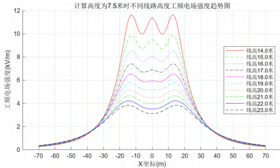
图 6.1-50 15mm 冰区单回水平线路距地面 7.5m 高处工频电场预测图
