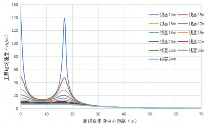
图 6.1-39 单回（水平排列）线路距地面 13.5m 高处工频电场预测图
