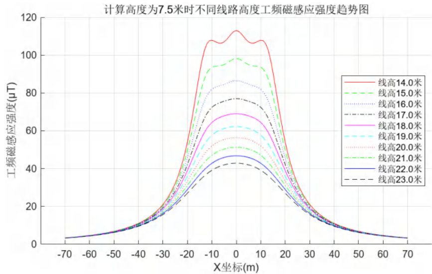
图 6.1-51 15mm 冰区单回水平线路距地面 7.5m 高处工频磁场预测图
