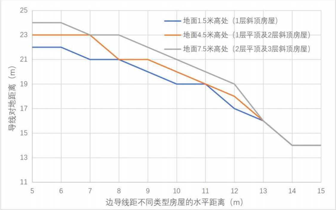
图 6.1-59 单回段路线不同高度处工频电场强度 4kV/m 等值线图
