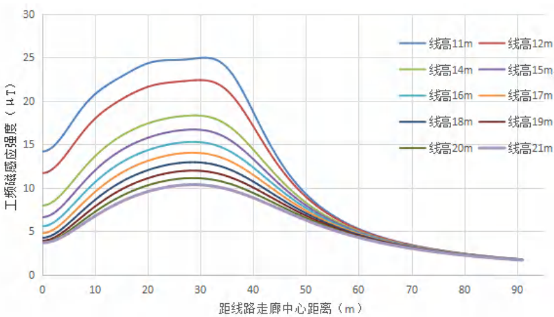
图 6.1-43 单回并行（水平排列）线路距地面 1.5m 高处工频磁场预测图
