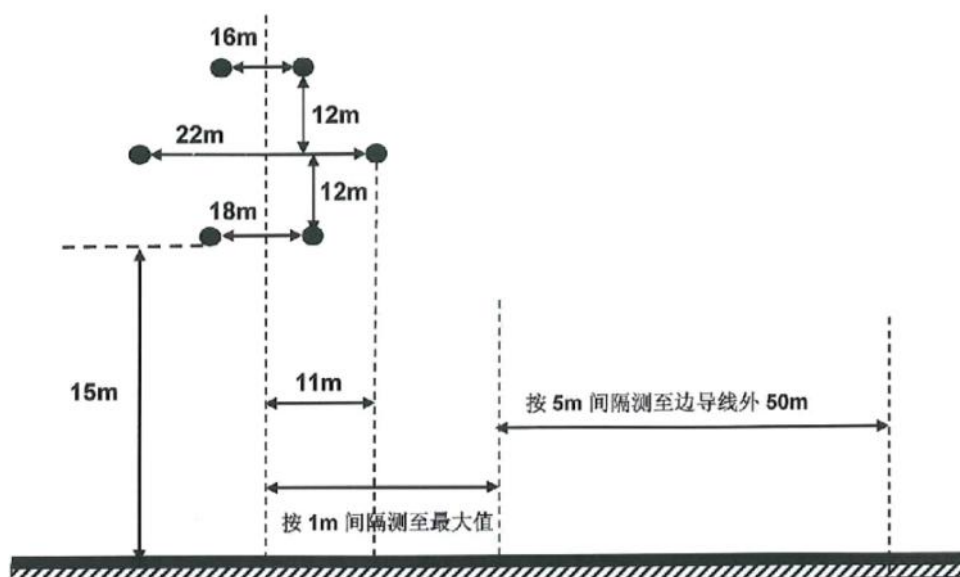
图 6.1-8 500kV 雁船 I、II 线同塔双回线路电磁环境监测断面示意图
