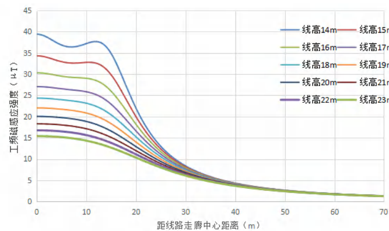
图 6.1-23 单回（水平排列）线路距地面 7.5m 高处工频磁场预测图
