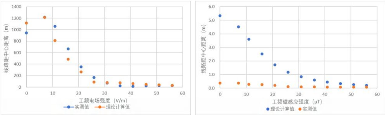
图 6.1-13 220kV 宗庄 I、II 线工频电场强度工频磁感应强度实测结果与理论计算结果对比图
