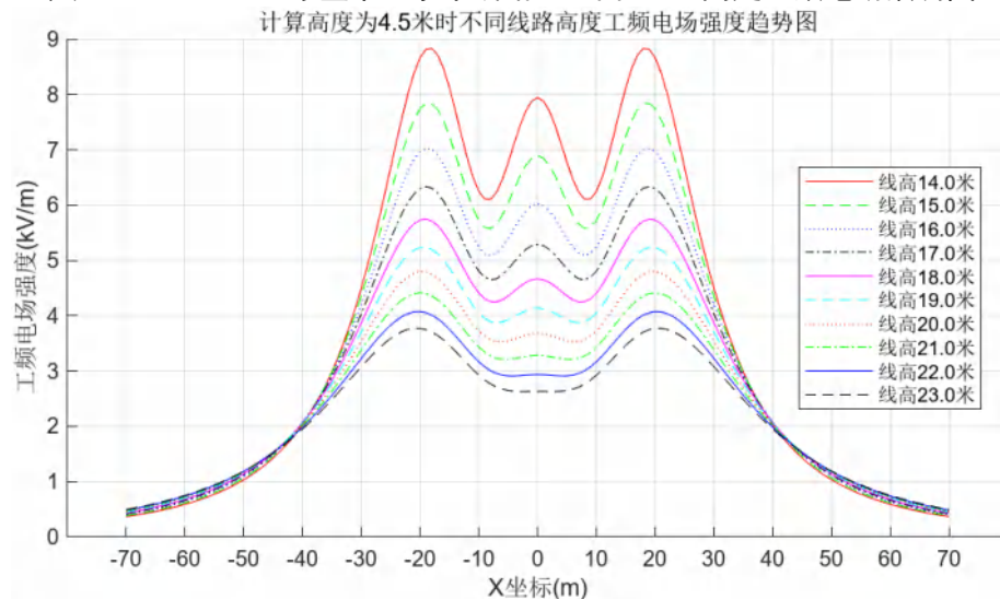
图 6.1-55 20mm 冰区单回水平线路距地面 4.5m 高处工频电场预测图
