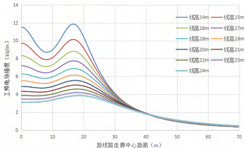
图 6.1-33 单回（水平排列）线路距地面 4.5m 高处工频电场预测图
