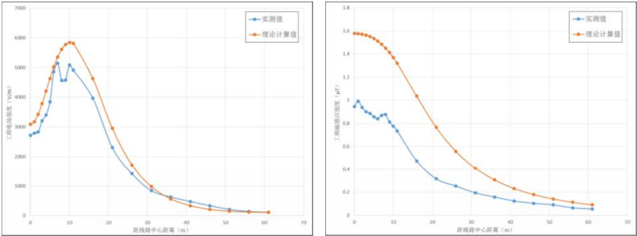
图 6.1-12 500kV 雁船 I、II 线工频电场强度、工频磁感应强度实测结果与理论计算结果对比图
