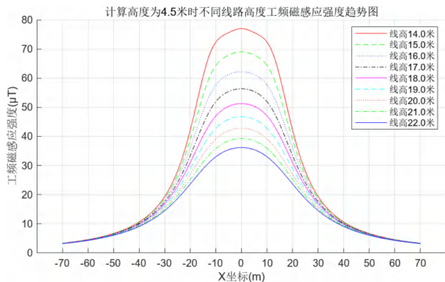
图 6.1-49 15mm 冰区单回水平线路距地面 4.5m 高处工频磁场预测图
