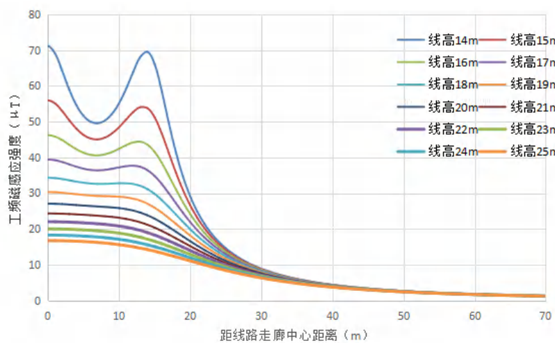
图 6.1-25 单回（水平排列）线路距地面 10.5m 高处工频磁场预测图
