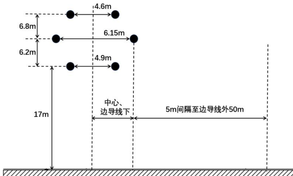
图 6.1-9 220kV 宗庄 I、II 线#11~#12 杆塔间电磁环境监测断面示意图
