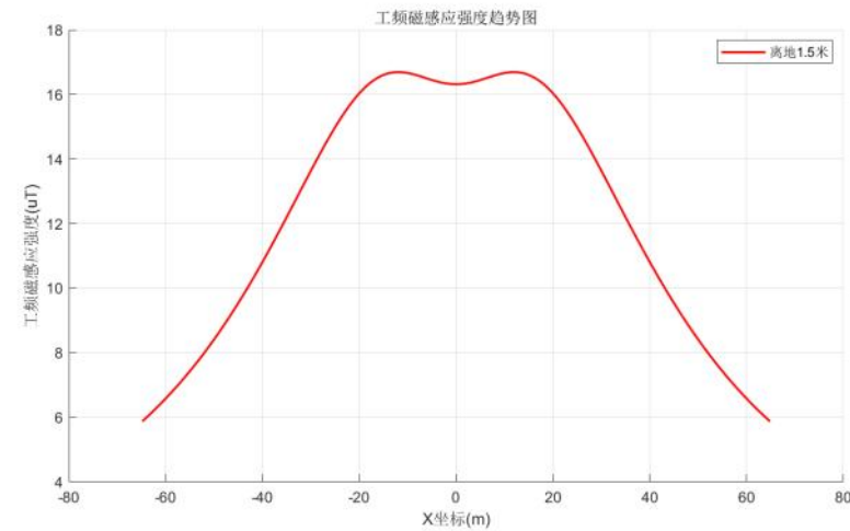
图 6.1-61 15mm 冰区双回共塔线路距地面 1.5m 高处工频磁场预测图（线高 27m）
