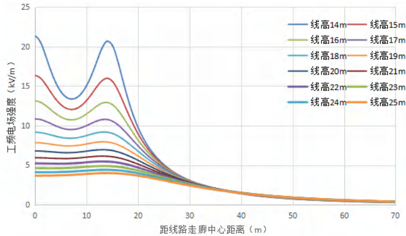
图 6.1-22 单回（水平排列）线路距地面 7.5m 高处工频电场预测图
