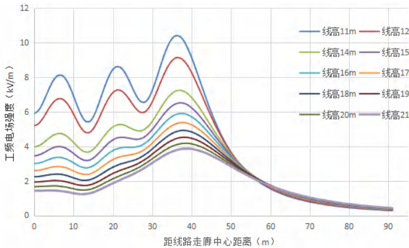
图 6.1-42 单回并行（水平排列）线路距地面 1.5m 高处工频电场预测图
