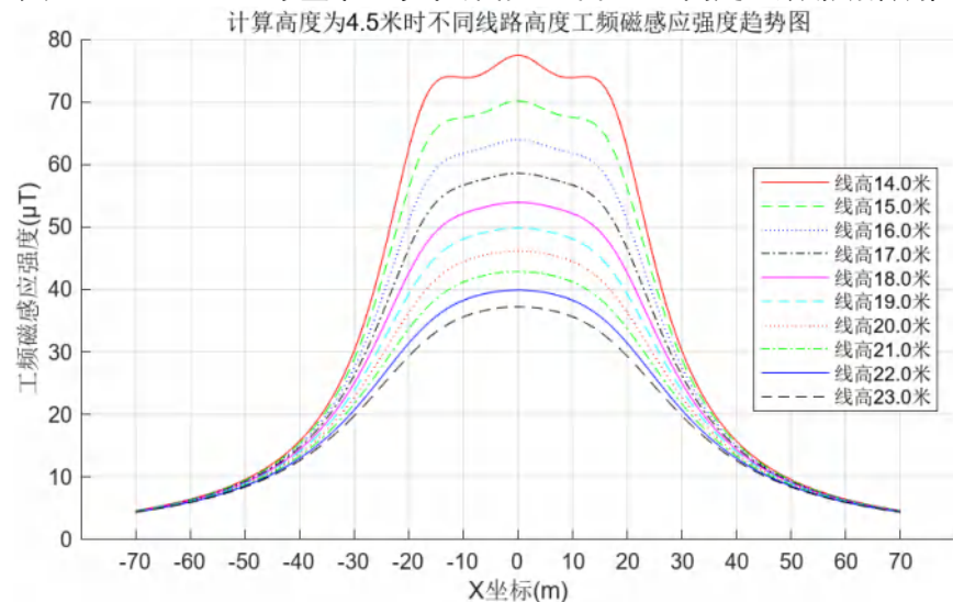
图 6.1-56 20mm 冰区单回水平线路距地面 4.5m 高处工频磁场预测图
