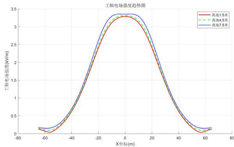
图 6.1-62 15mm 冰区双回共塔线路距地面 1.5m、4.5m、7.5m 高处工频电场预测图（线高 29m）
