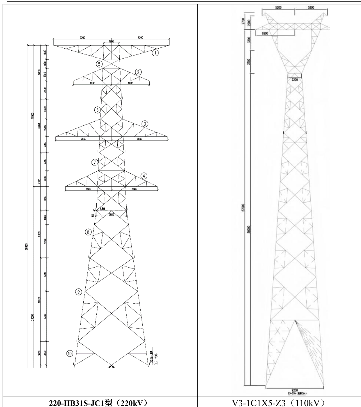
图 6.1-17 本项目 220kV 和 110kV 线路电磁环境预测选择的代表性塔型图
