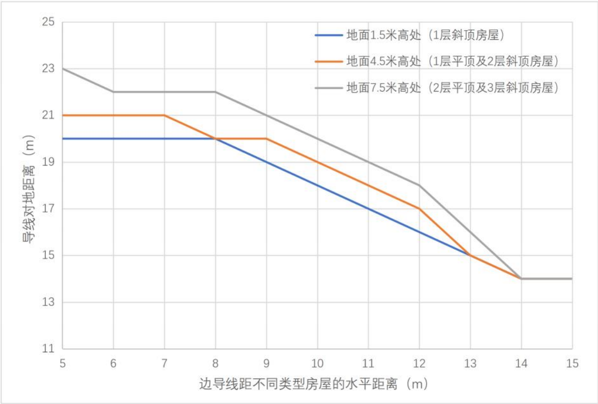
图 6.1-52 单回路路线不同高度处工频电场强度 4kV/m 等值线图
