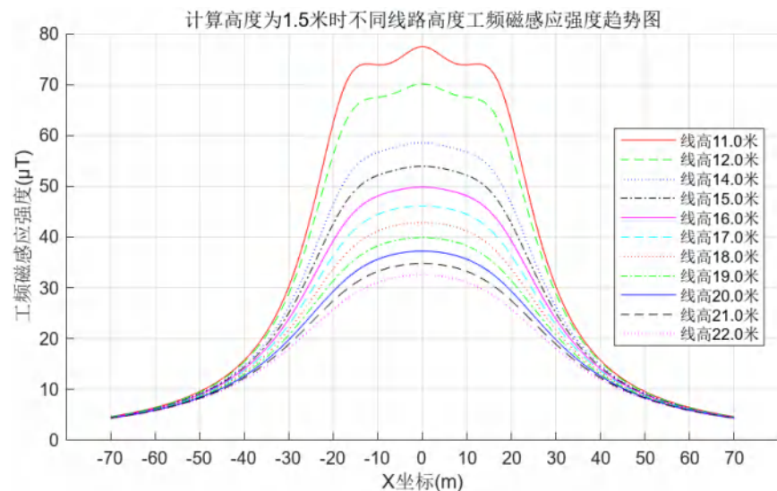
图 6.1-54 20mm 冰区单回水平线路距地面 1.5m 高处工频磁场预测图
