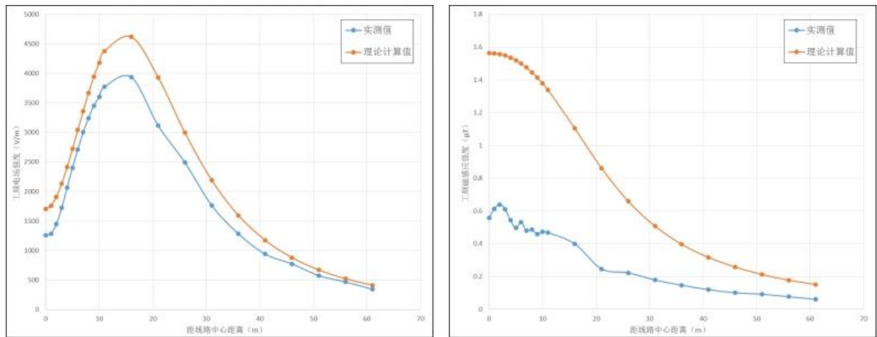
图 6.1-11 500kV 雁船 II 线工频电场强度、工频磁感应强度实测结果与理论计算结果对比图
