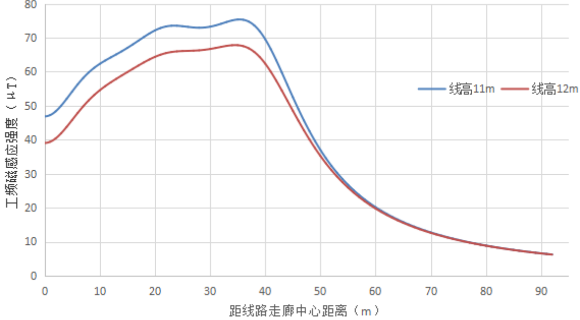
图 6.1-45 单回并行（水平排列）线路距地面 1.5m 高处工频磁场预测图
