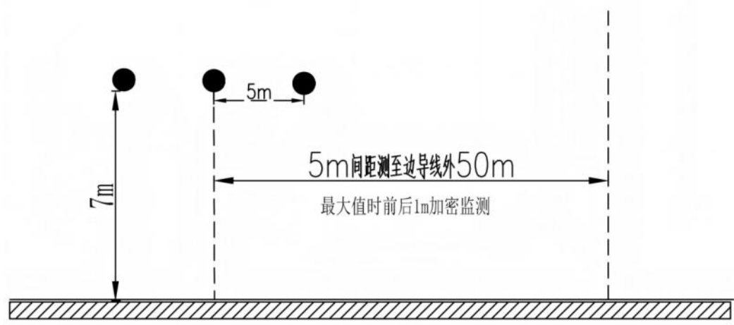
图 6.1-10 110kV 杨东线新建 13#~14#塔间线电磁环境监测断面示意图 类比监测期间运行工况情况见下表。
