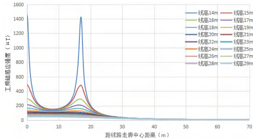
图 6.1-40 单回（水平排列）线路距地面 13.5m 高处工频磁场预测图
