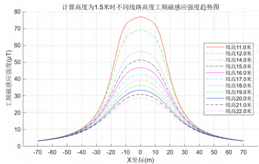
图 6.1-47 15mm 冰区单回水平线路距地面 1.5m 高处工频磁场预测图
