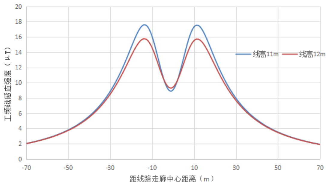
图 6.1-30 500kV 同塔双回线路距地面 1.5m 高处工频磁场预测图
