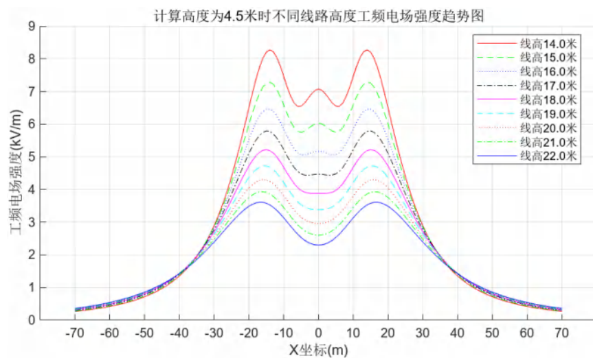
图 6.1-48 15mm 冰区单回水平线路距地面 4.5m 高处工频电场预测图
