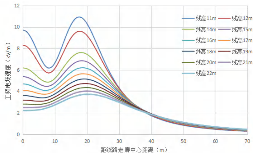
图 6.1-31 单回（水平排列）线路距地面 1.5m 高处工频电场预测图
