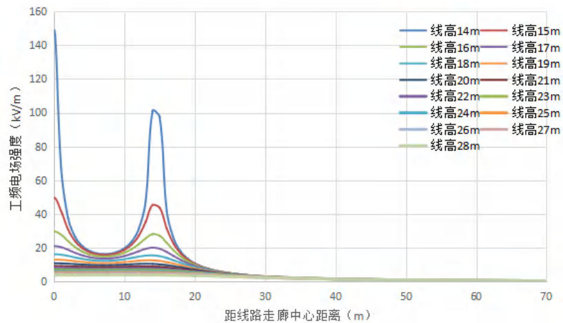
图 6.1-26 单回（水平排列）线路距地面 13.5m 高处工频电场预测图
