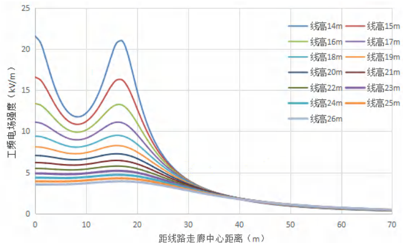
图 6.1-37 单回（水平排列）线路距地面 10.5m 高处工频电场预测图
