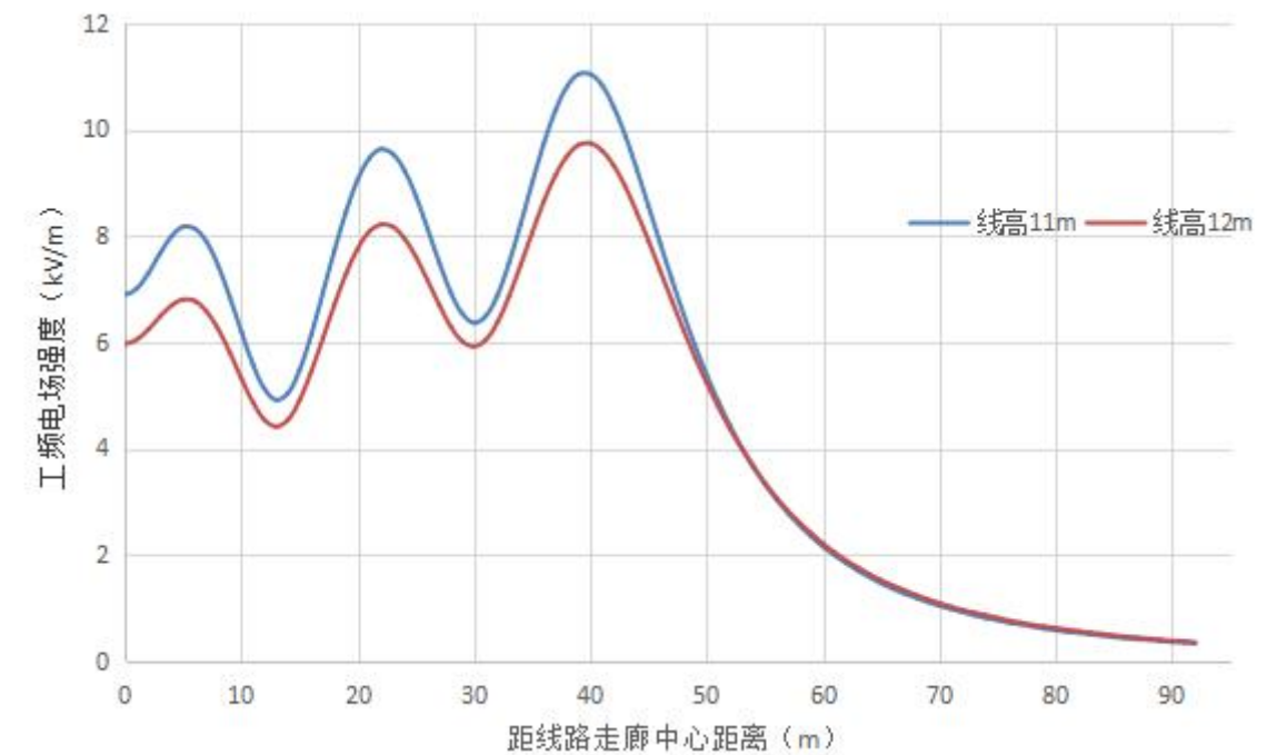
图 6.1-44 单回并行（水平排列）线路距地面 1.5m 高处工频电场预测图
