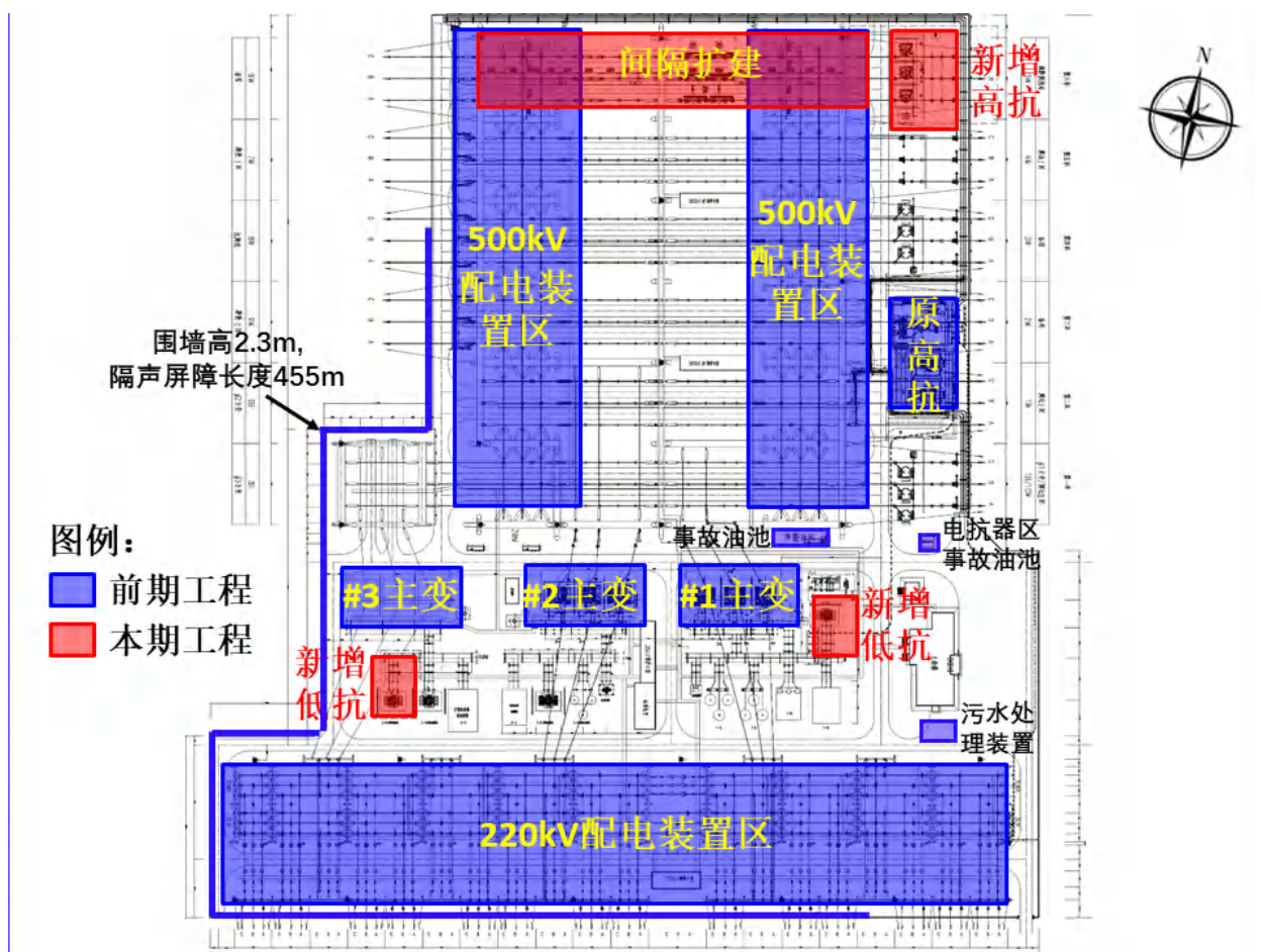
图 3.1-8 牌楼 500kV 变电站平面布置示意图
