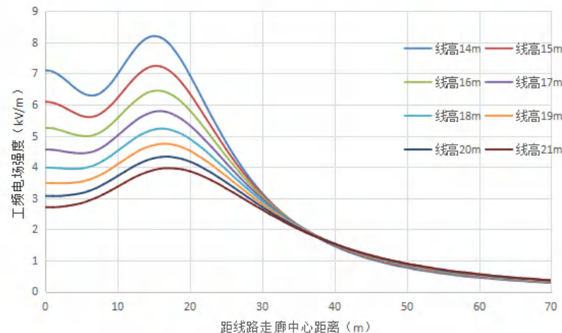
图 6.1-20 单回（水平排列）线路距地面 4.5m 高处工频电场预测图
