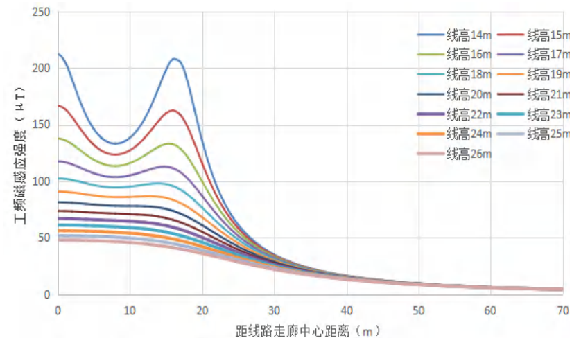
图 6.1-38 单回（水平排列）线路距地面 10.5m 高处工频磁场预测图
