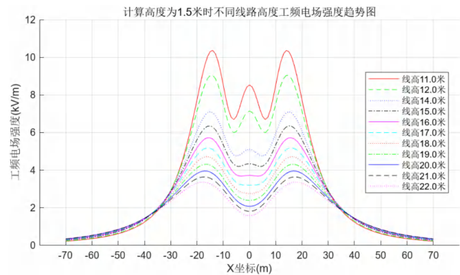
图 6.1-46 15mm 冰区单回水平线路距地面 1.5m 高处工频电场预测图
