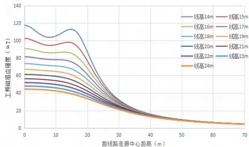
图 6.1-36 单回（水平排列）线路距地面 7.5m 高处工频磁场预测图
