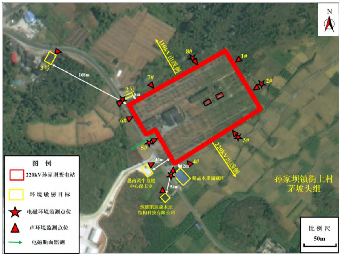
图 6.1-6 类比孙家坝 220kV 变电站电磁监测布点示意图
