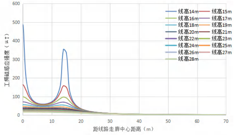
图 6.1-27 单回（水平排列）线路距地面 13.5m 高处工频磁场预测图
