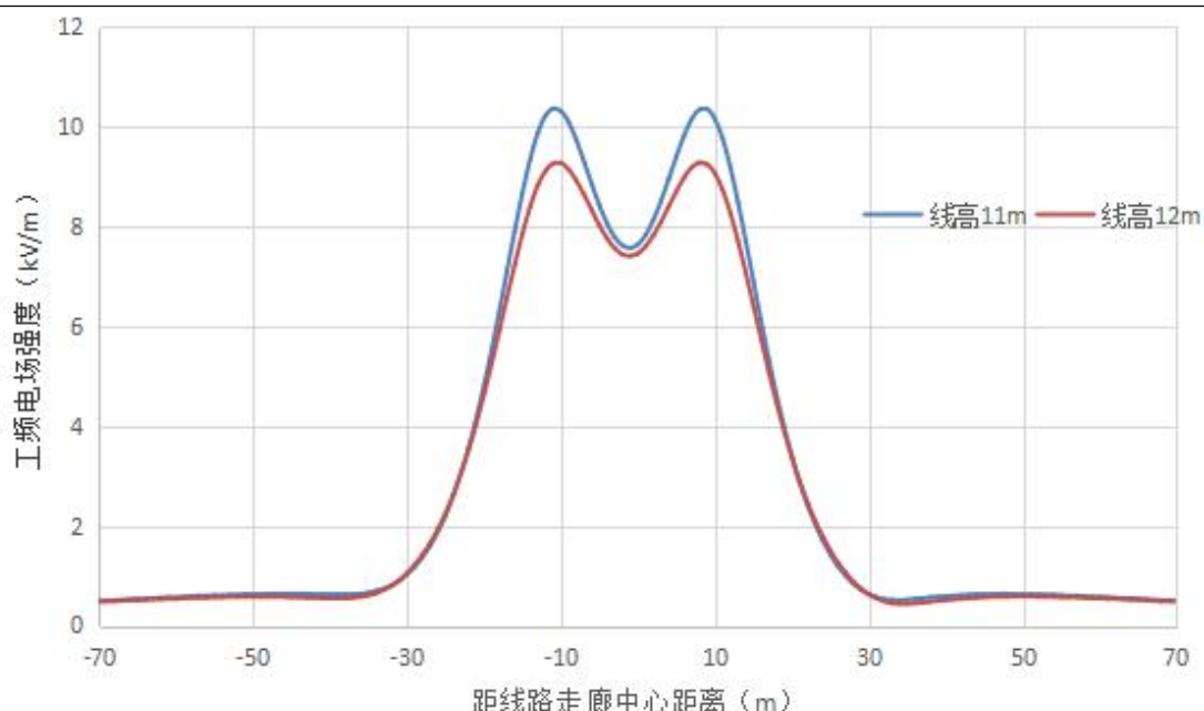
图 6.1-29 500kV 同塔双回线路距地面 1.5m 高处工频电场预测图
