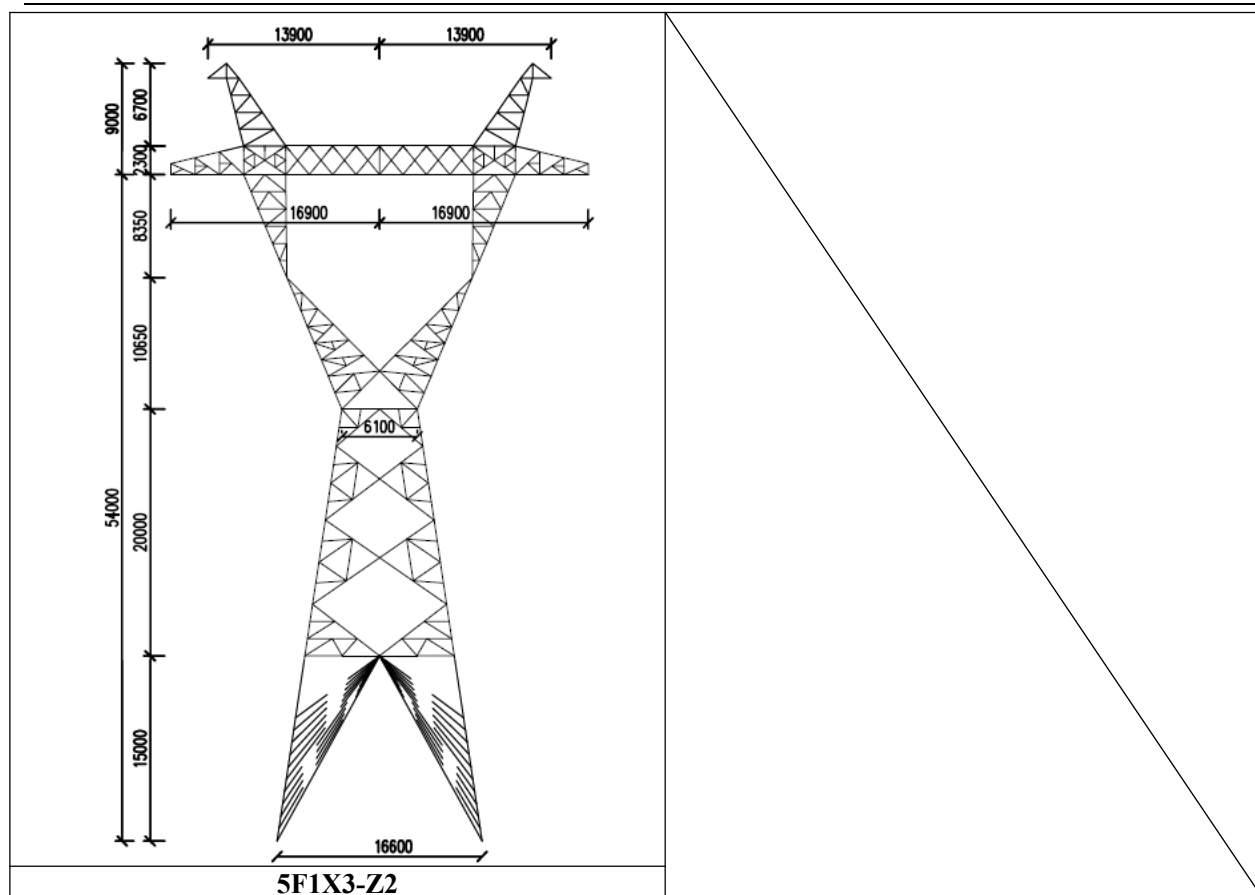
图 6.1-15 本项目 500kV 线路（贵州段）电磁环境预测选择的代表性塔型图
