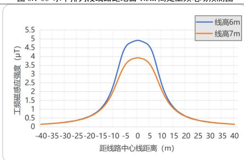
图 6.1-67 水平排列线路距地面 1.5m 高处工频磁场预测图
