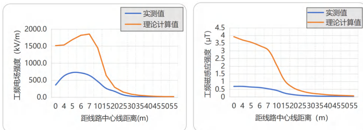
图 6.1-14 本项目 110kV 线路（水平排列）工频电场强度工频磁感应强度实测结果与理论计算结果对比图
