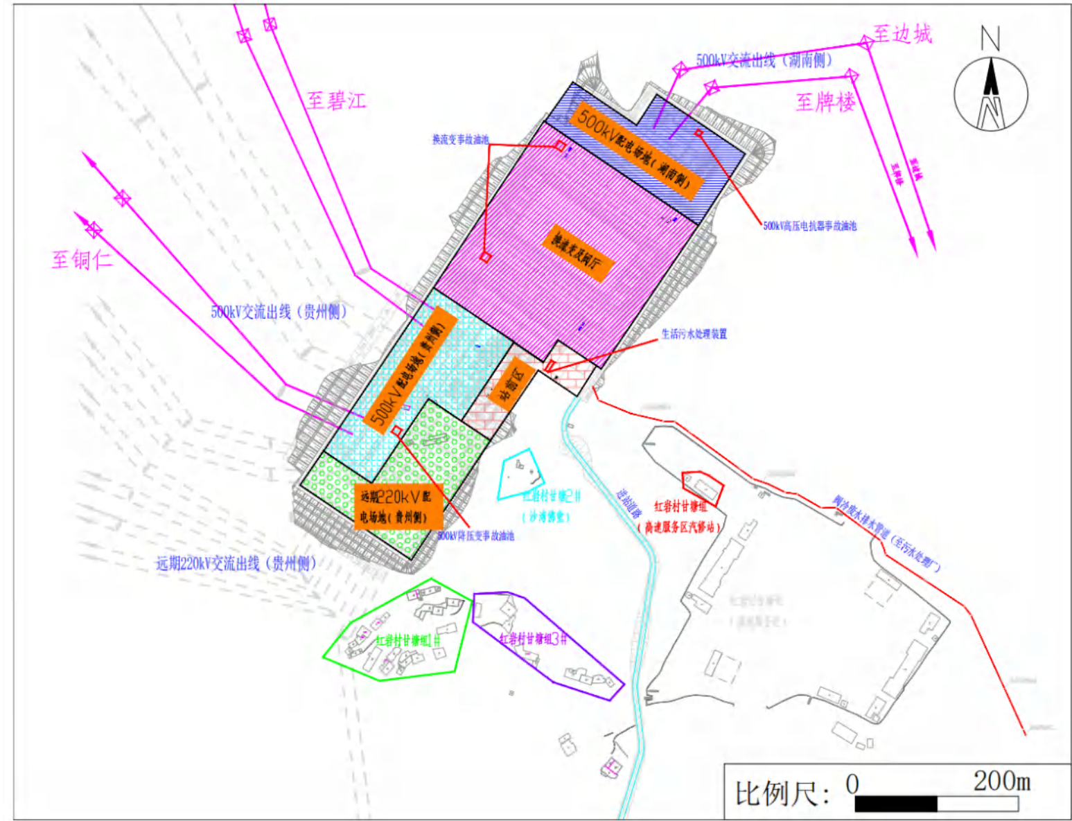
图 3.1-2 本项目换流站总平面布置图
