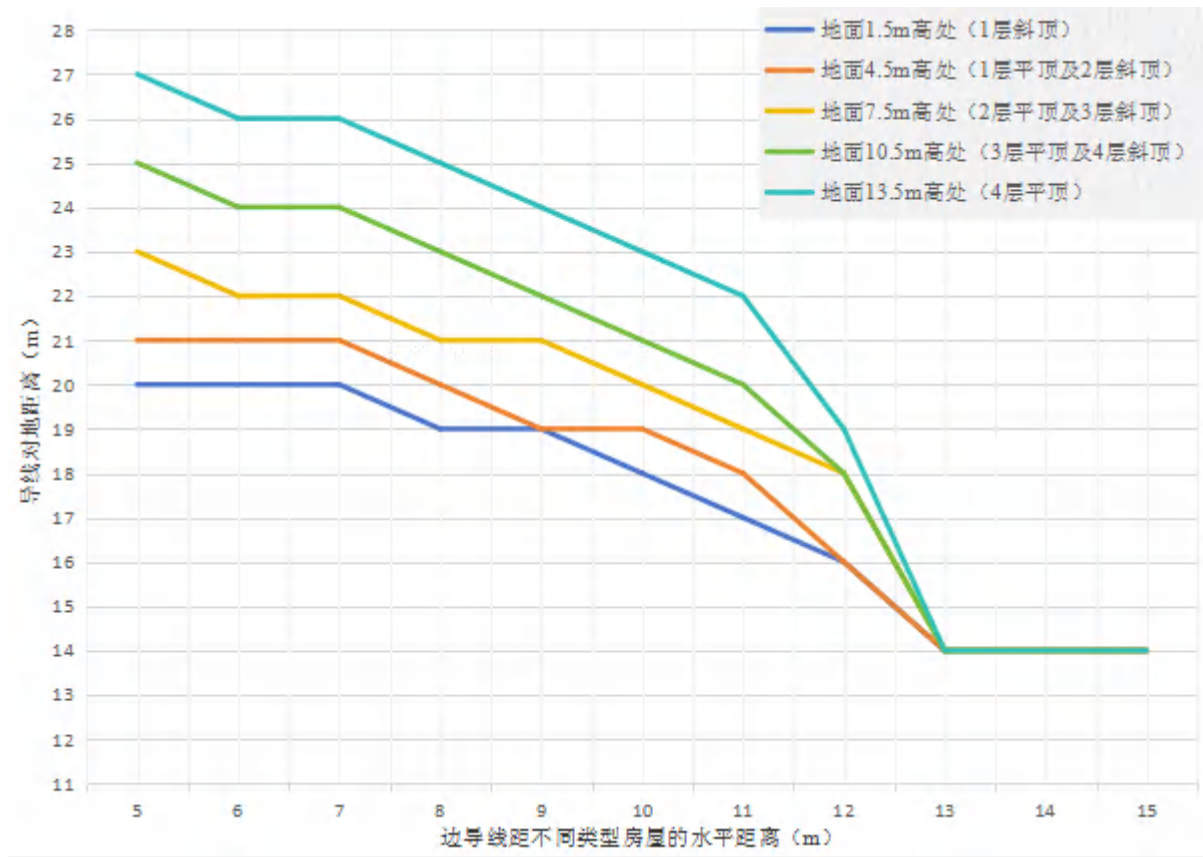
图 6.1-28 500kV 线路单回线路（水平排列）路线不同高度处工频电场强度 4kV/m 等值线图
